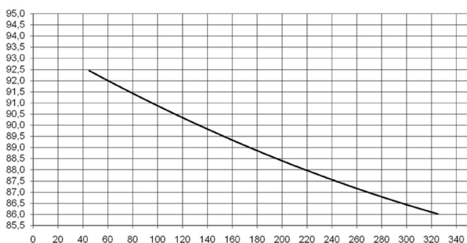
Courbe rendement
