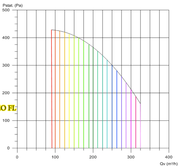
Courbe aéralique
